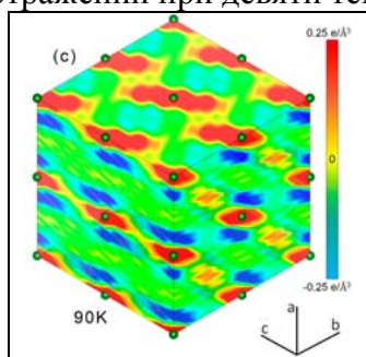
Рис. 1. Формирование системы проводящих каналов в GdB_6 , 90K
