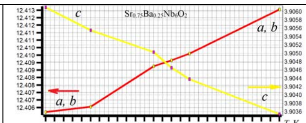
Рис. 2. Зависимость параметров ячейки a, b, c от температуры, есть слабая особенность 296 К.
