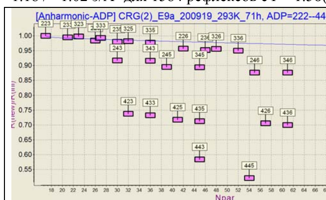
Рис. 1. Оценка значимости расширения ангармонической модели смещения атомов. N_{\text{par}} – число параметров модели. R_{\text{new}} / R_{\text{ini}} – отношение R -факторов для расширенной модели к R -фактору начальной модели
