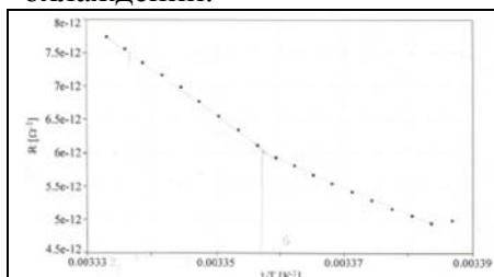
Рис. 1. Зависимость сопротивления от температуры имеет излом при 297.7 К
